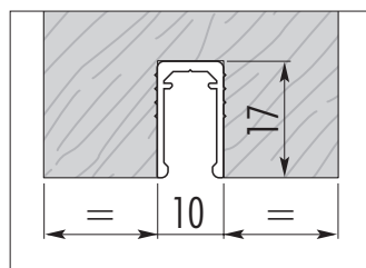
Detail vsunutého ochranného profilu
