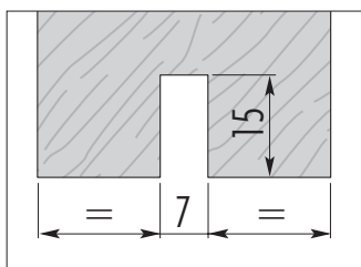
Detail vyfrézovaného dveřního křídla
